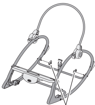
8 Retainers with Lock Nut Retenedores con tuerca ciega Dispositifs de retenue avec contre-écrou Contentores com trava
