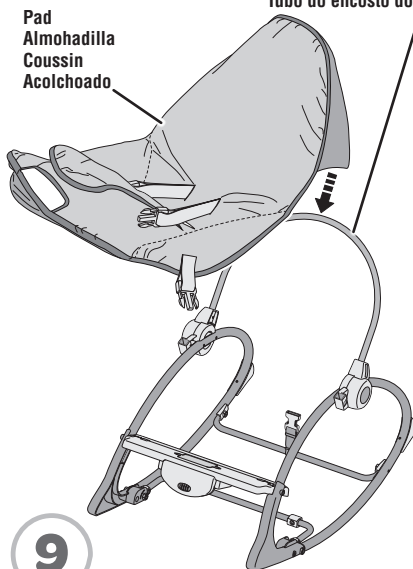
Seat Back Tube Tubo del respaldo Tube du dossier Tubo do encosto do assento
