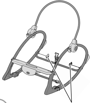
Retainers with Lock Nut Retenedores con tuerca ciega
