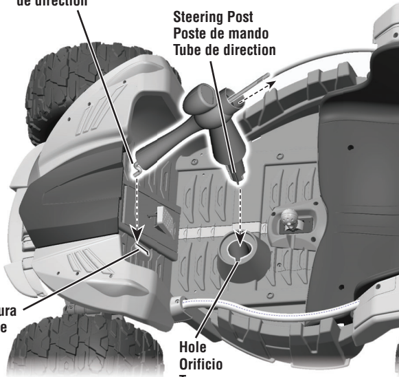
TOP SIDE VIEW VISTA LATERAL DE ARRIBA VUE DE DESSUS
