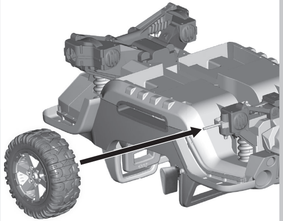
Front Wheel Rueda delantera Roue avant
