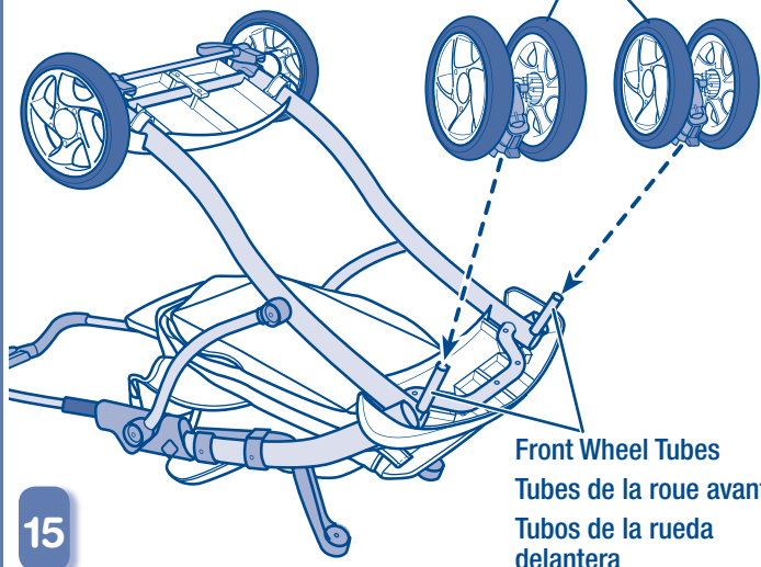
Front Wheel Assemblies Assemblages de roue avant Unidades de rueda delantera
