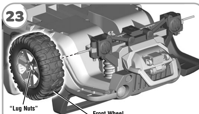
Front Wheel Rueda delantera Roue avant
