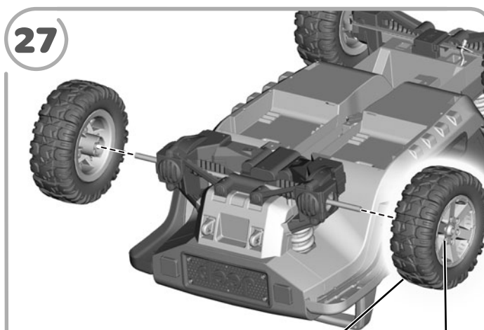
Rear Wheel Rueda trasera Roue arrière "Lug Nuts" "Orejeras" Verrous
