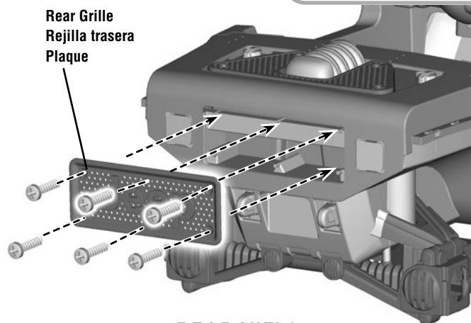
REAR VIEW VISTA DESDE ATRÁS VUE DE L'ARRIÈRE
