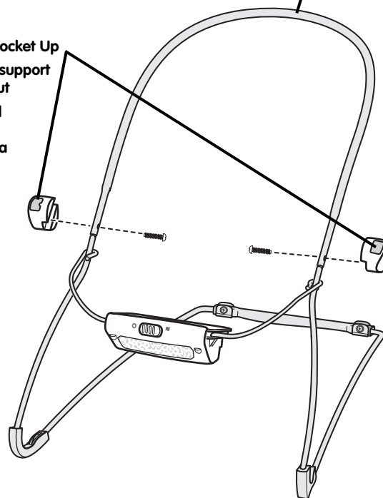
Seat Back Tube Tube du dossier Tubo del respaldo
