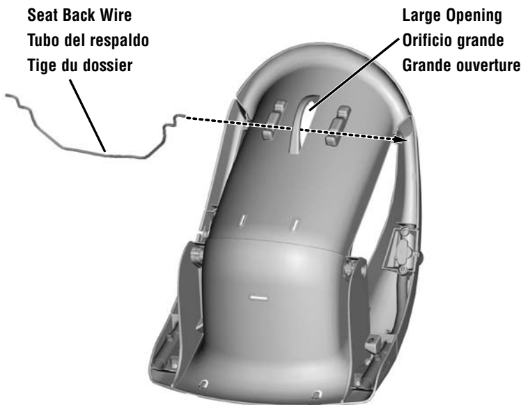
BOTTOM VIEW VISTA DESDE ABAJO VUE DE DESSOUS
