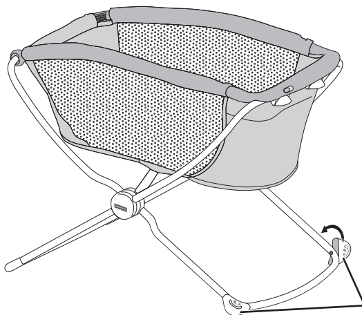
Locking Feet Patas bloqueadoras Pieds verrouillables Pés de travamento
