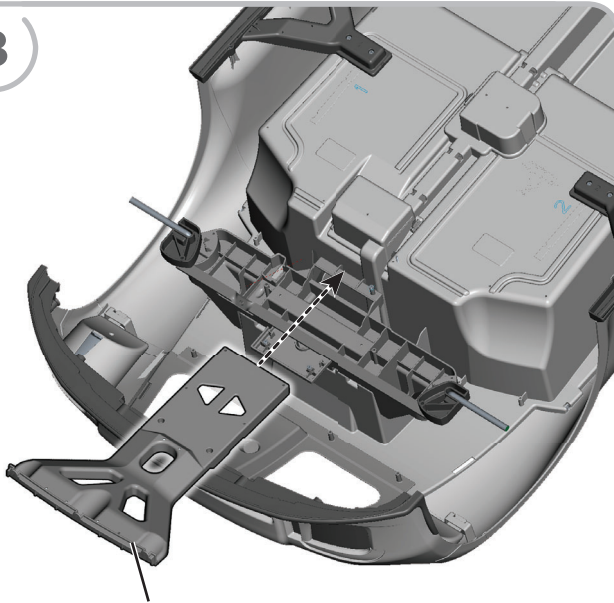
Front Bumper Support Soporte de la defensa delantera Support à pare-chocs
