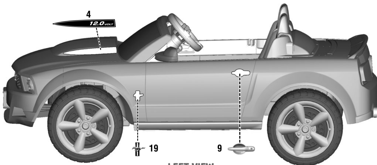
LEFT VIEW VISTA DE LA IZQUIERDA VUE DU CÔTÉ GAUCHE
