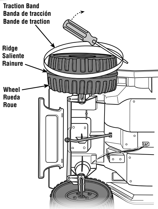
BOTTOM VIEW VISTA DESDE ABAJO VUE DE DESSOUS
