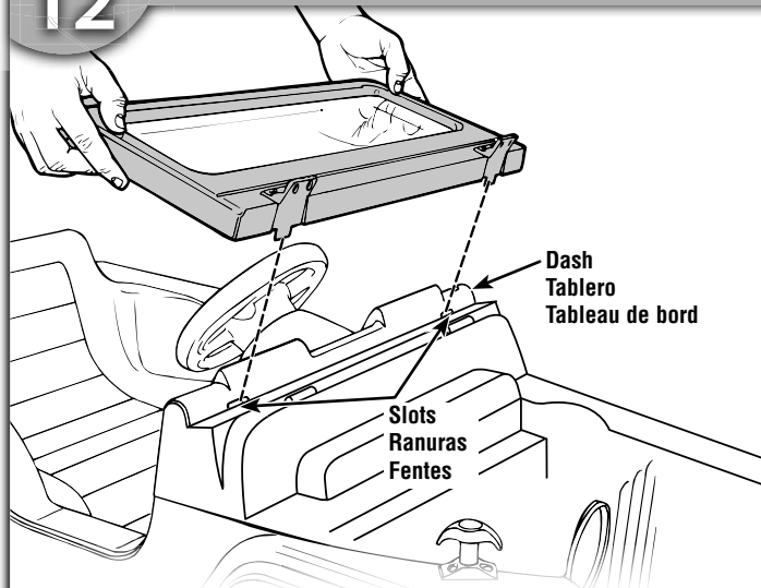
FRONT SIDE VIEW VISTA FRONTAL LATERAL VUE DE L'AVANT
